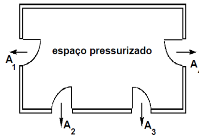
Figura 1 - Trajetórias de escape do ar em paralelo
