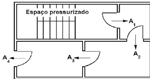
Figura 2 - Trajetórias de escape do ar em série
