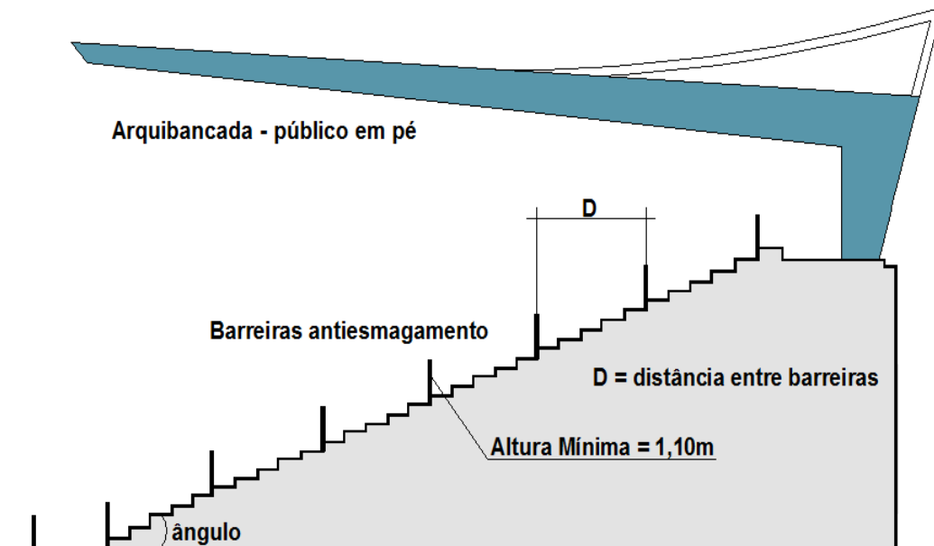
Resistência mecânica e distâncias entre barreiras antiesmagamentos
