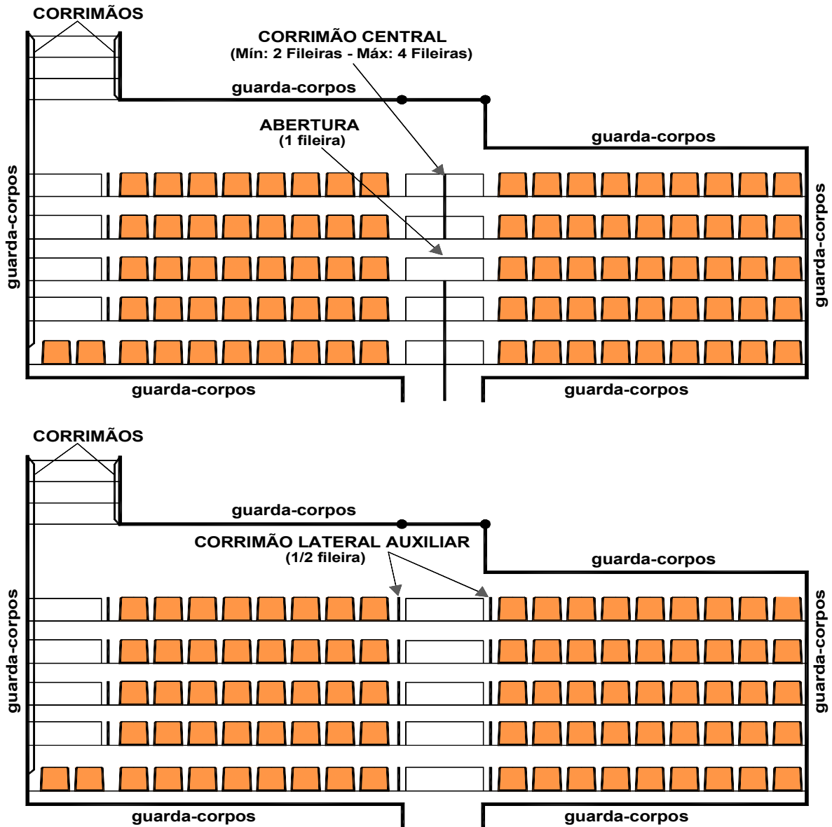
Figura 6 Corrimãos centrais e laterais
