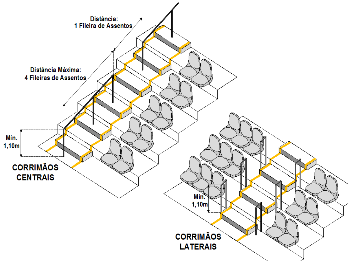
Figura 12 Perspectiva de corrimãos centrais e laterais
