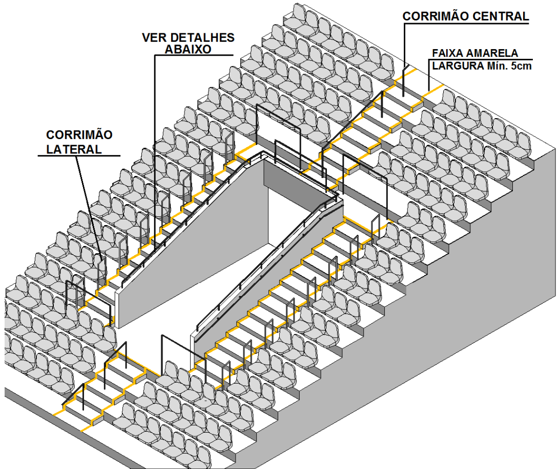
Figura 11 Perspectiva de vomitório padrão
