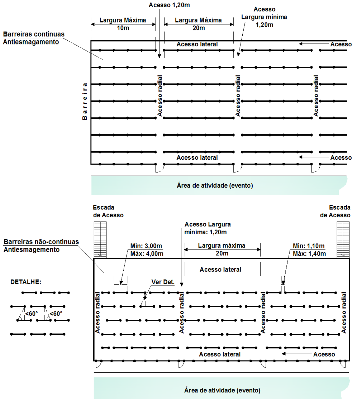
Figura 10 Barreiras antiesmagamento – contínuas e não-contínuas
