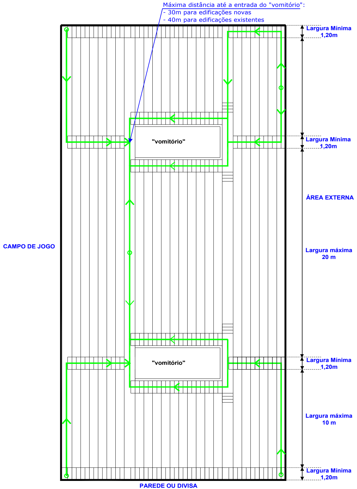
Figura 8 Distâncias a percorrer e acessos
