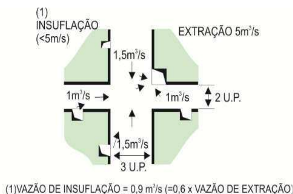
Figura 28 - Resumo geral de aberturas de extração de fumaça e entrada de ar em um pavimento
