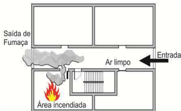
Figura 21 -Extração natural
