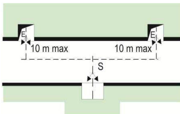
Figura 25 - Distância em linha reta de aberturas de extração
