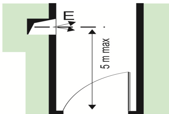
Figura 27 - Distância de introdução de ar de portas de acesso
