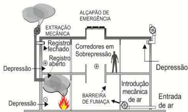
Figura 23 - Controle por sobrepressão
