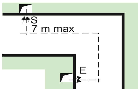
Figura 26 - Distância de extração de aberturas em trajeto diversos
