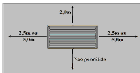
Figura 3 – Distâncias mínimas de aberturas à tomada de ar
