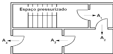
Figura 2 - Trajetórias de escape do ar em série
