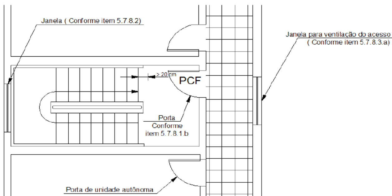
Figura 8 — Ventilação da escada enclausurada protegida e seu acesso
