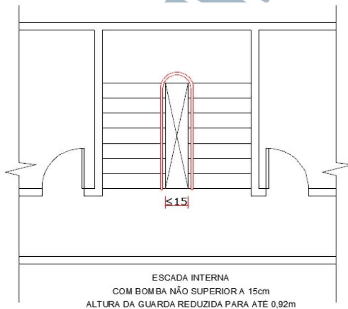
Figura 27 - Escada interna com bomba não superior a 0,15m
