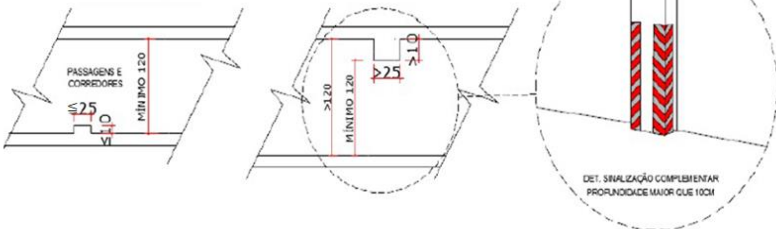
Figura 1 - Medida da largura em corredores e passagens
