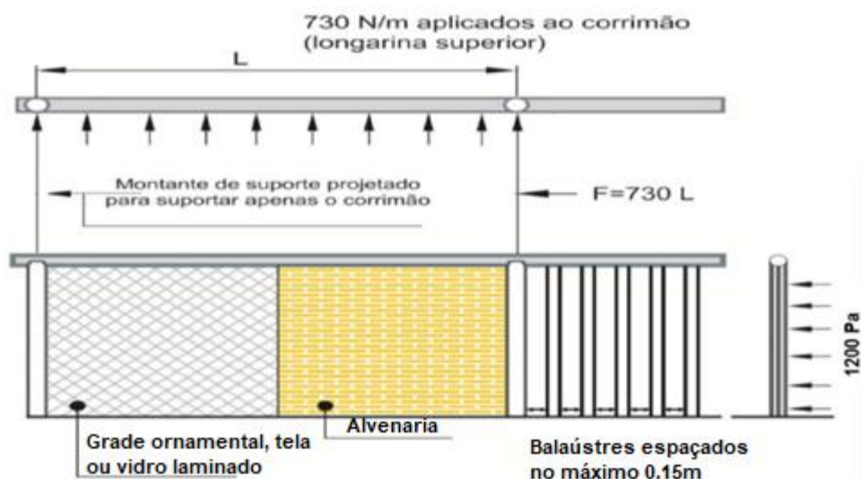
Figura 32 – Pormenores construtivos da instalação de guardas e as cargas a que elas devem resistir
