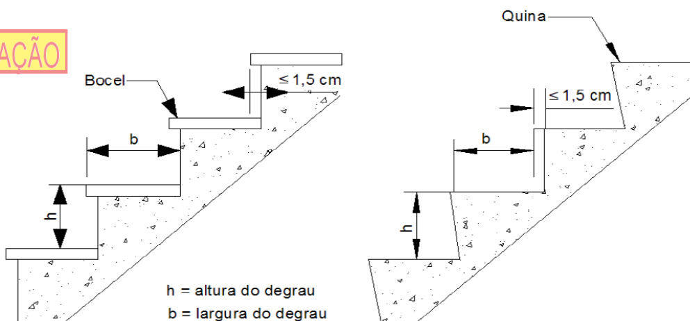
Figura 13 – Altura e largura dos degraus
