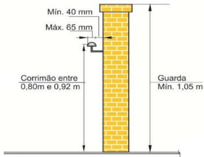
Figura 14 – Dimensões do guardas e corrimãos
