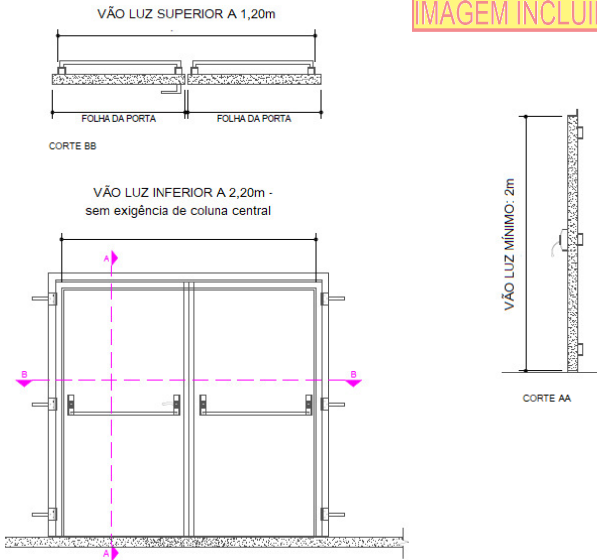
Figura 7- Porta corta-fogo em duas folhas
