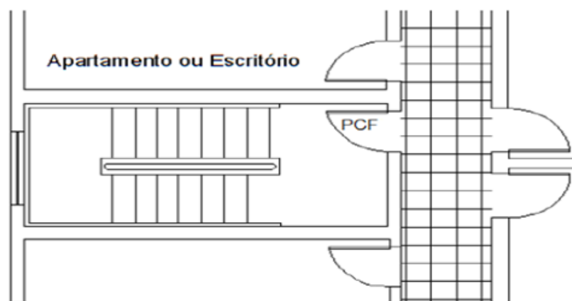
Figura 7 — Escada enclausurada protegida Figura 19 — Escada enclausurada protegida
