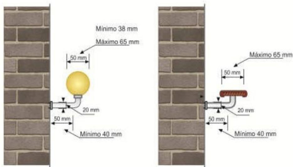
Figura 15 — Pormenores de corrimãos
