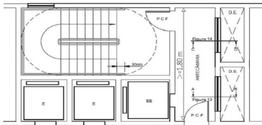
Figura 9 – Escada enclausurada à prova de fumaça com elevador de emergência na antecâmara
