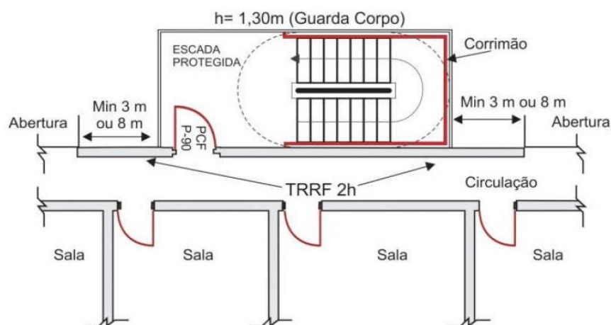
Figura 12 — Escada aberta externa
