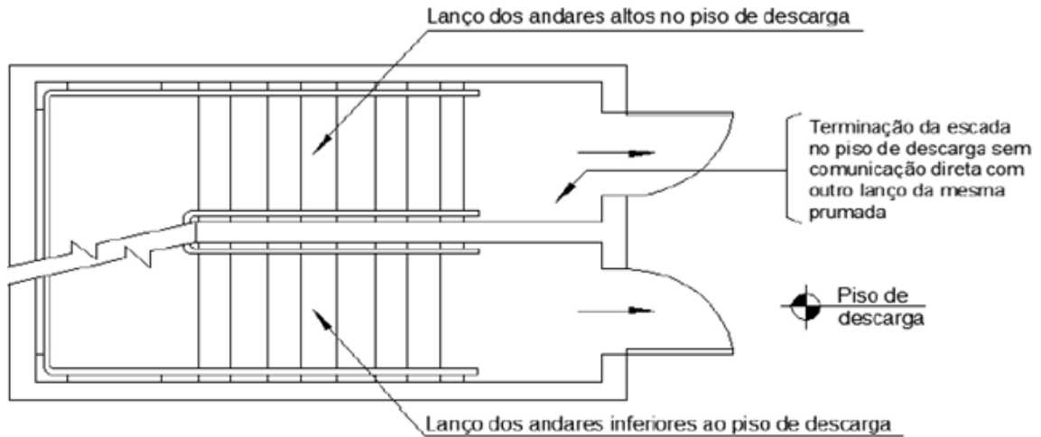
Figura 3 – Segmentação das escadas no piso de descarga Figura 9 – Segmentação das escadas no piso de descarga
