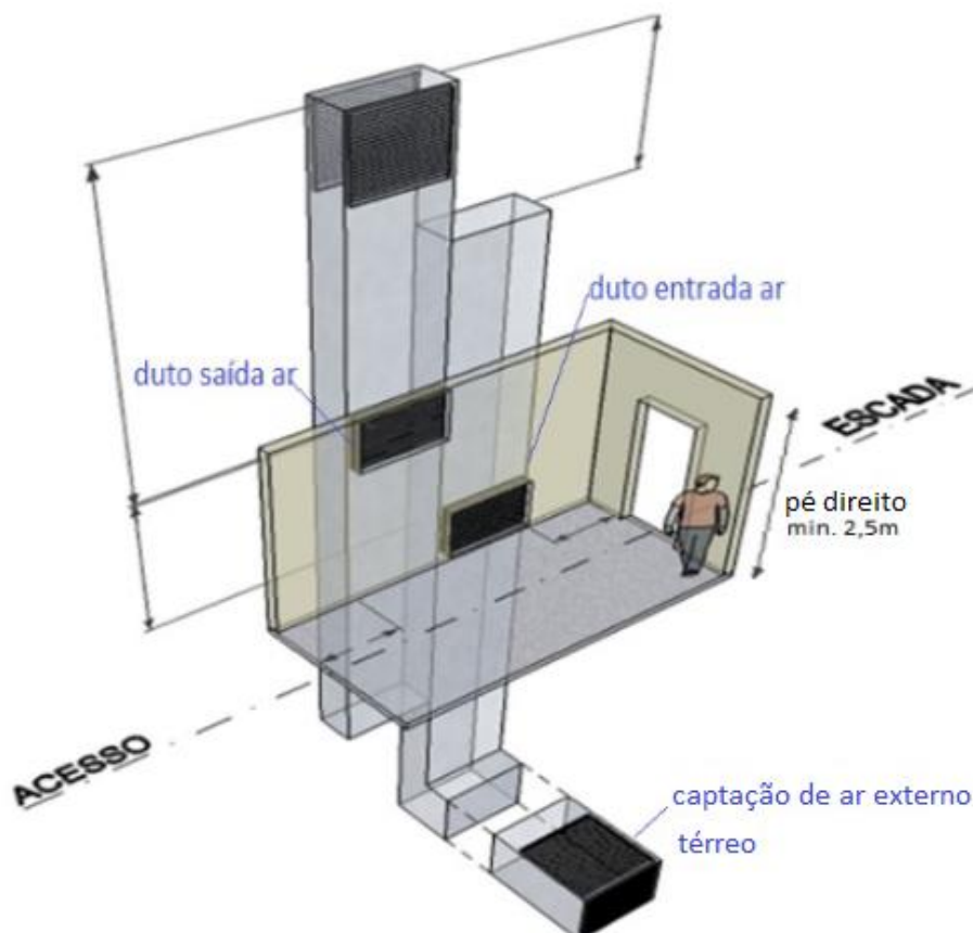
Figura 10 – Dutos de entrada e saída de ar
