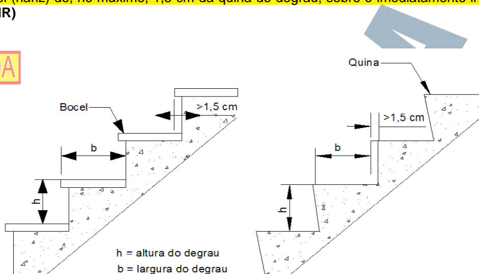
Figura 4 — Altura e largura dos degraus
