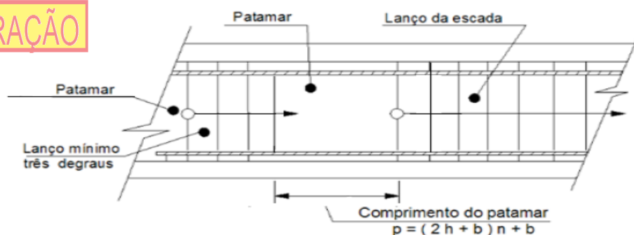
Figura 15 - Lanço mínimo e comprimento de patamar
