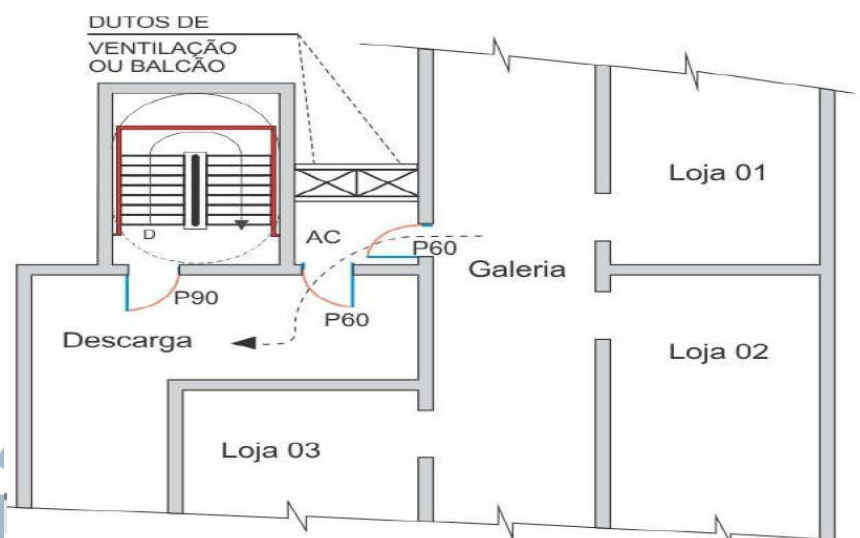
Figura 20 – Acesso de galeria comercial à descarga Figura 36 - Acesso de galeria comercial à descarga
