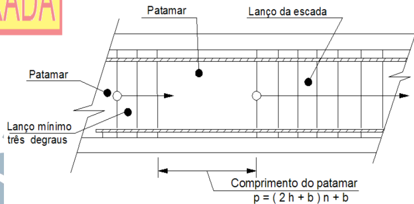
Figura 6 — Lanço mínimo e comprimento de patamar
