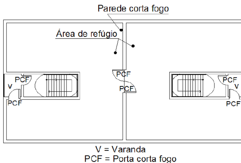
Figura 17 – Desenho esquemático da área de refúgio Figura 33 – Desenho esquemático da área de refúgio
