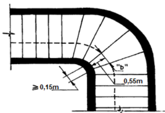
Figura 5 — Escada com lanços curvos e degraus balanceados. Figura 14 — Escada com lanços curvos e degraus balanceados
