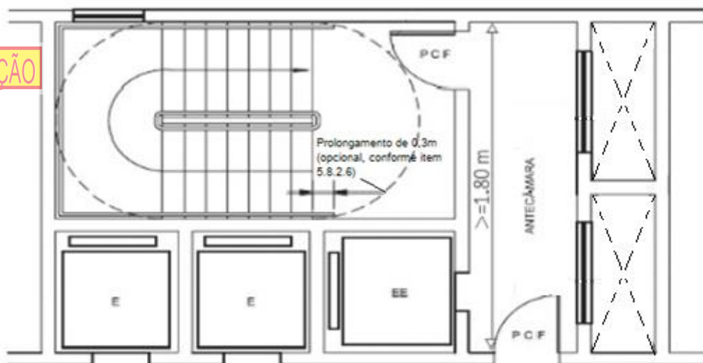
Figura 21 – Escada enclausurada à prova de fumaça com elevador de emergência na antecâmara
