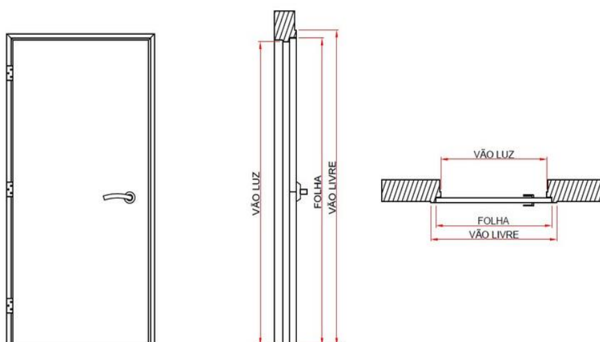
Figura 6 - Portas corta fogo: identificação de vão luz e vão livre
