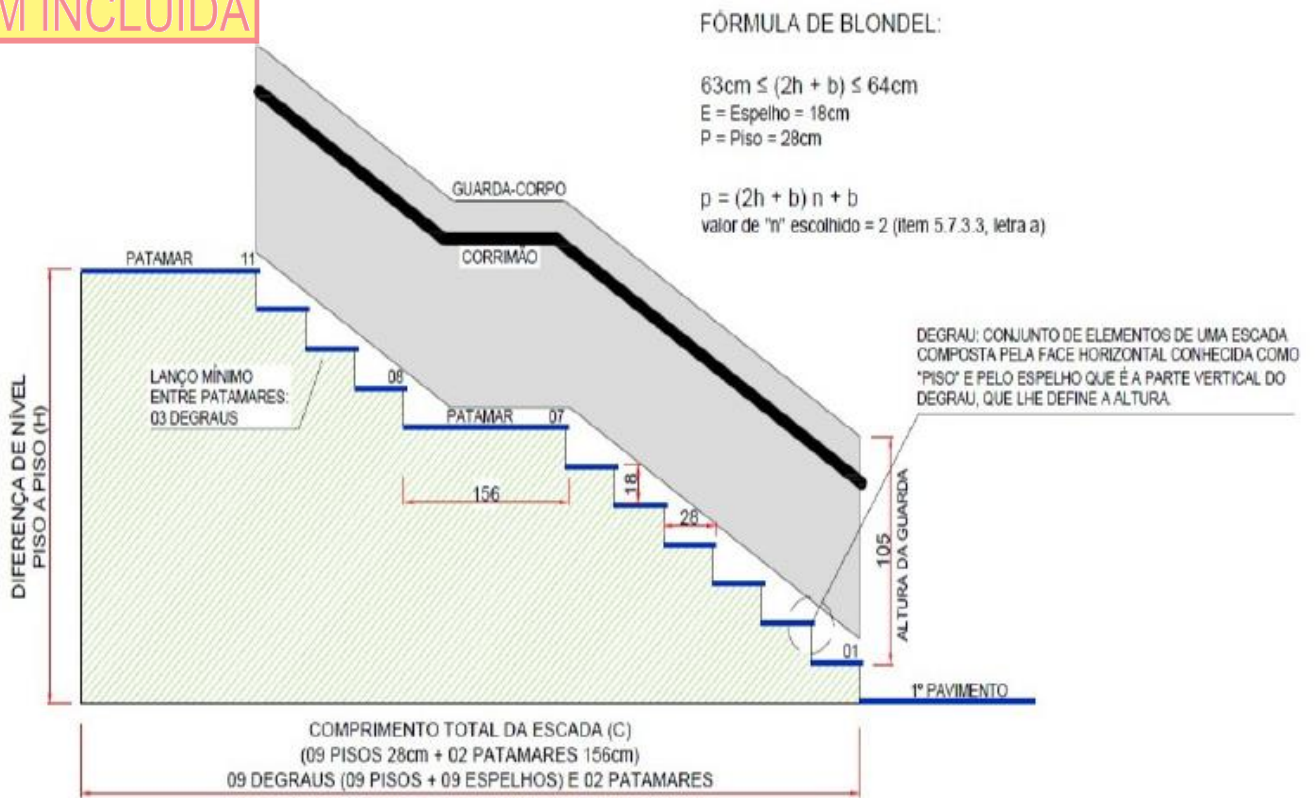
Figura 16 - Exemplo de dimensionamento
