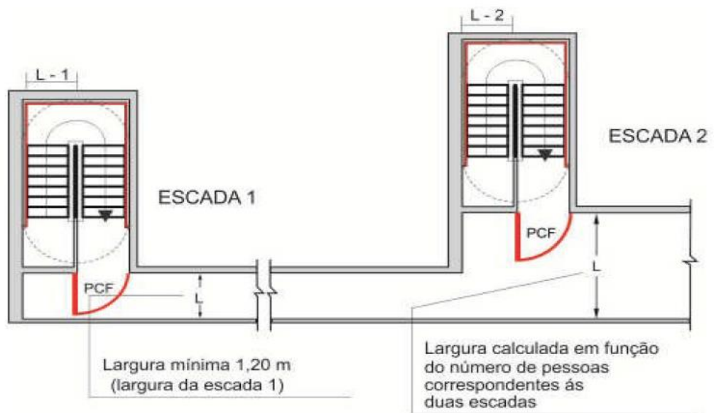
Figura 19 – Dimensionamento de corredores de descarga Figura 35 – Dimensionamento de corredores de descarga
