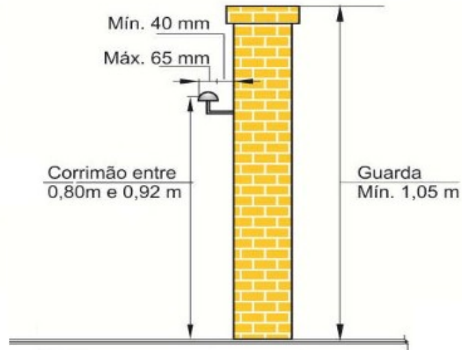
Figura 26 - Guarda-corpo de escada externa com altura não superior a 12 m ou escadas internas com bomba superior a 0,15 m
