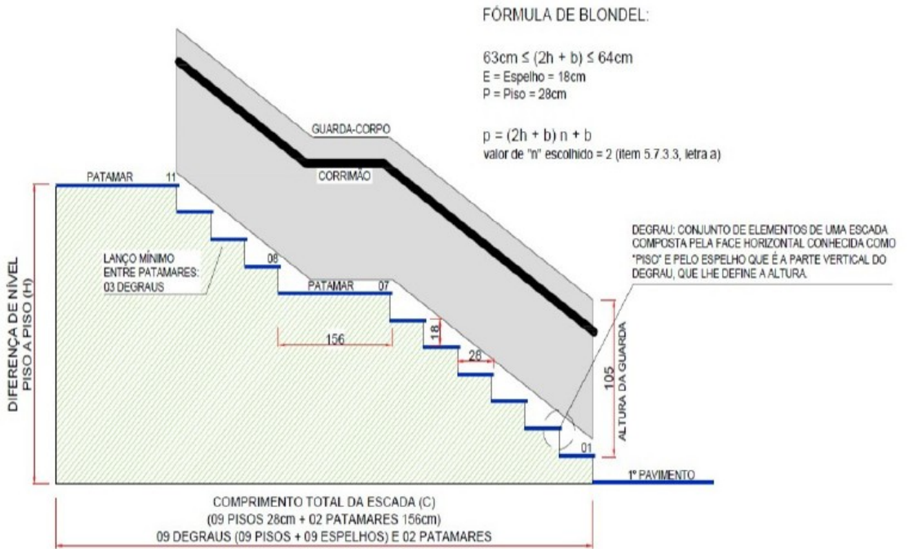
Figura 16 - Exemplo de dimensionamento
