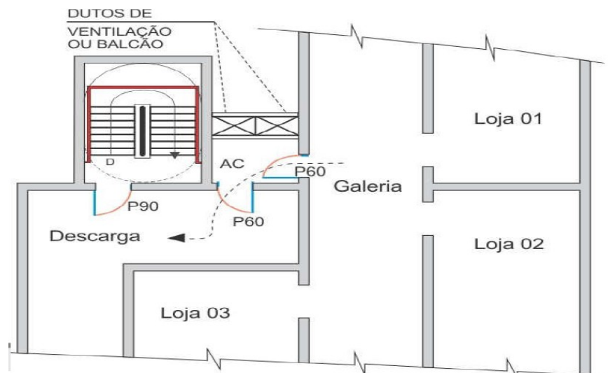
Figura 35 - Acesso de galeria comercial à descarga
