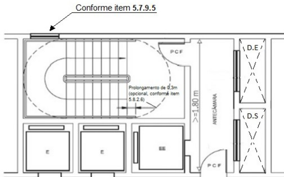
Figura 21 – Escada enclausurada à prova de fumaça com elevador de emergência na antecâmara
