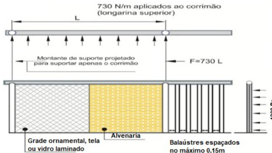
Figura 31 – Pormenores construtivos da instalação de guardas e as cargas a que elas devem resistir
