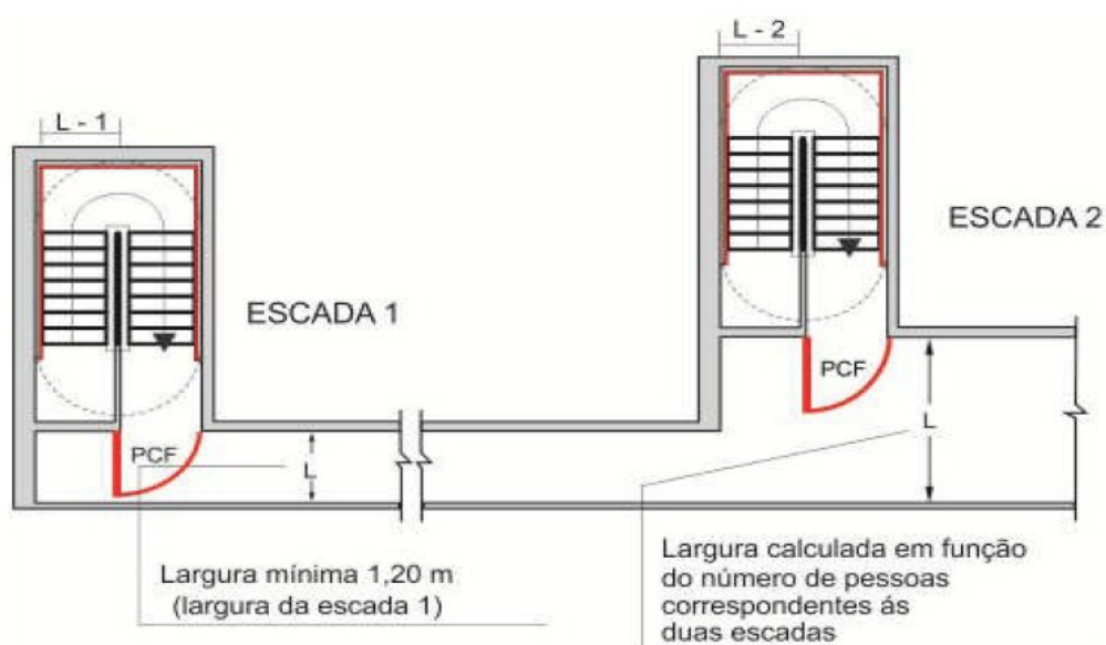
Figura 34 – Dimensionamento de corredores de descarga
