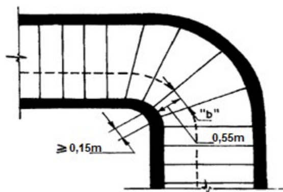
Figura 14 – Escada com lanços curvos e degraus balanceados
