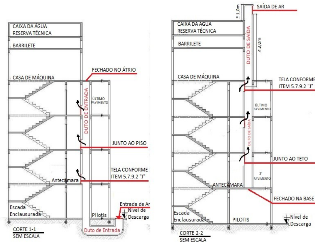
Figura 22-A – Exemplos de dutos de ventilação
