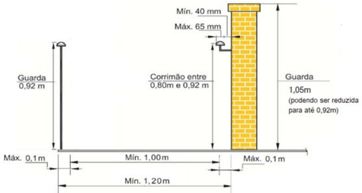
Figura 28 - Guarda-corpo de escada interna com bomba não superior a 0,15 m
